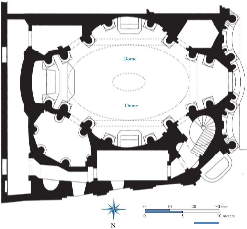
19-10 FRANCESCO BORROMINI, plan of San Carlo alle Quattro Fontane, Rome, Italy, 1638–1641.
